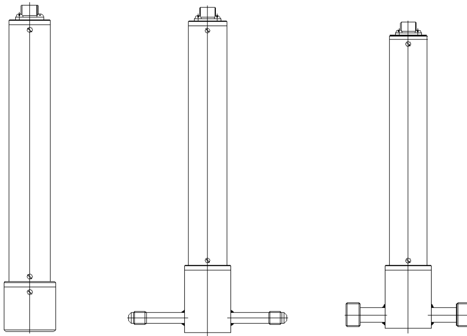
Рисунок 3.15 Измерительные преобразователи объемной доли кислорода ИПК-01, ИПК-01-М8, ИПК-01-М16 (по порядку слева направо)
