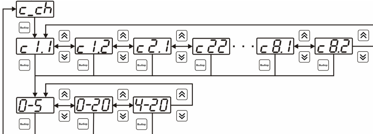
Рисунок 6.17 Настройка входного параметра канала управления (токовый)
